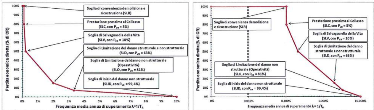
Figura 1– Andamento della curva che individua il PAM, riferito a una costruzione con vita nominale 50 anni e appartenente alla classe d'uso II. Nell'immagine a destra, per meglio individuare i punti prossimi all'asse delle ordinate, le ascisse sono in scala logaritmica.
